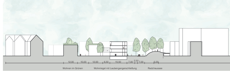
Schnitt 1-1
