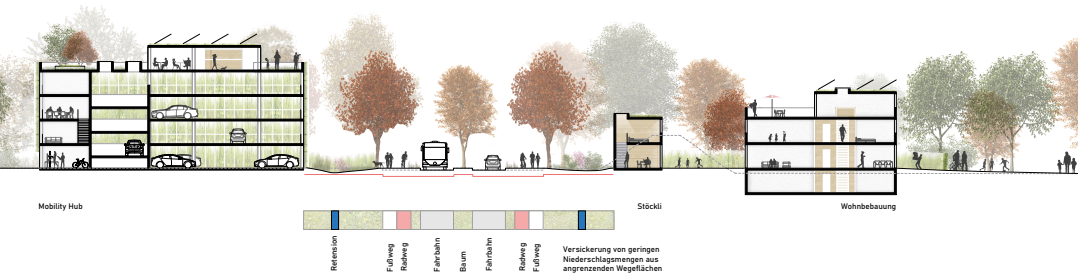
SCHNITTE M 1:200
